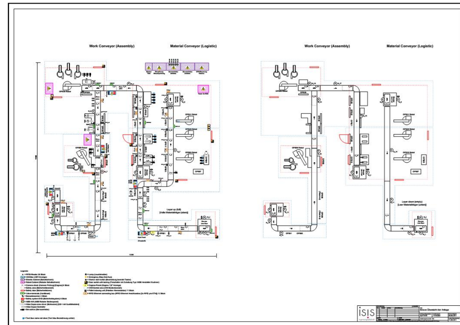
• Anlagenübersicht
