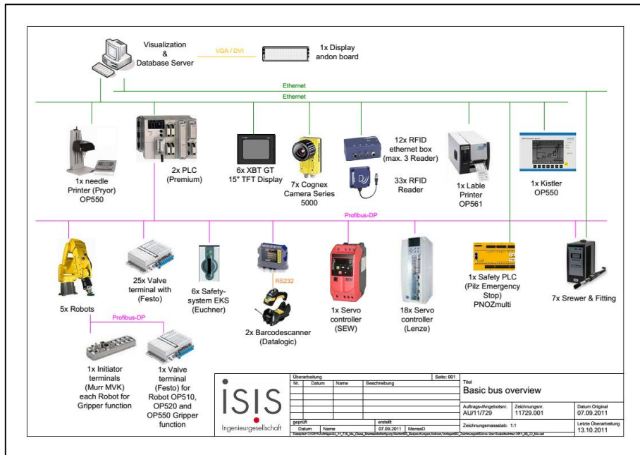
• Busteilnehmerübersicht
